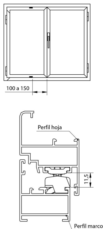
COLOCACIÓN Y ESQUEMA DE MONTAJE
