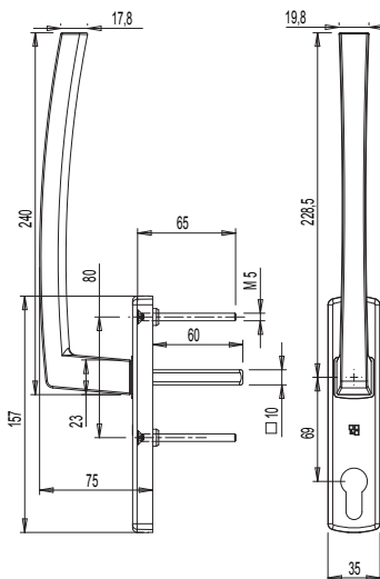
Dimensiones martelina ASIA L240 KEY -I80
