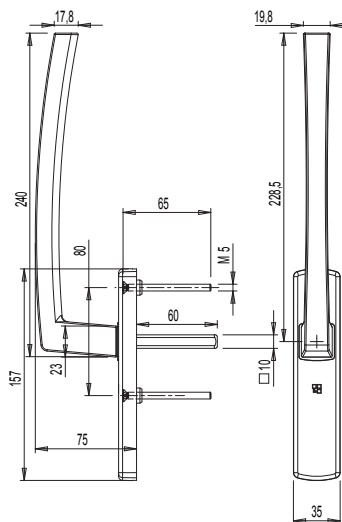
Dimensiones martelina ASIA L240 -I80
